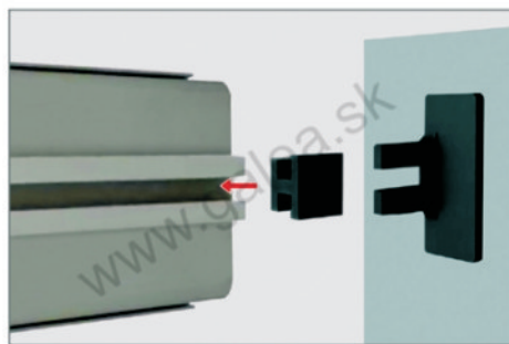
umiestnenie protikusu k úchytu S346
